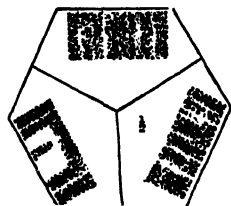
Calcite.
